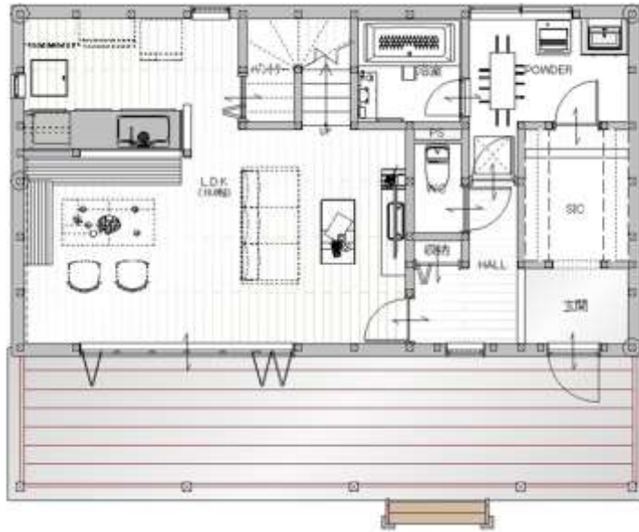
サニーサイドハウスⅢ 平面図 (1F)
