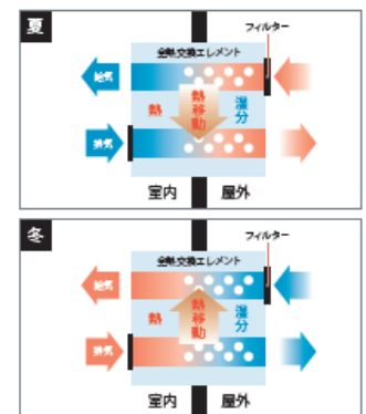
【全熱交換型換気システム概念図】
